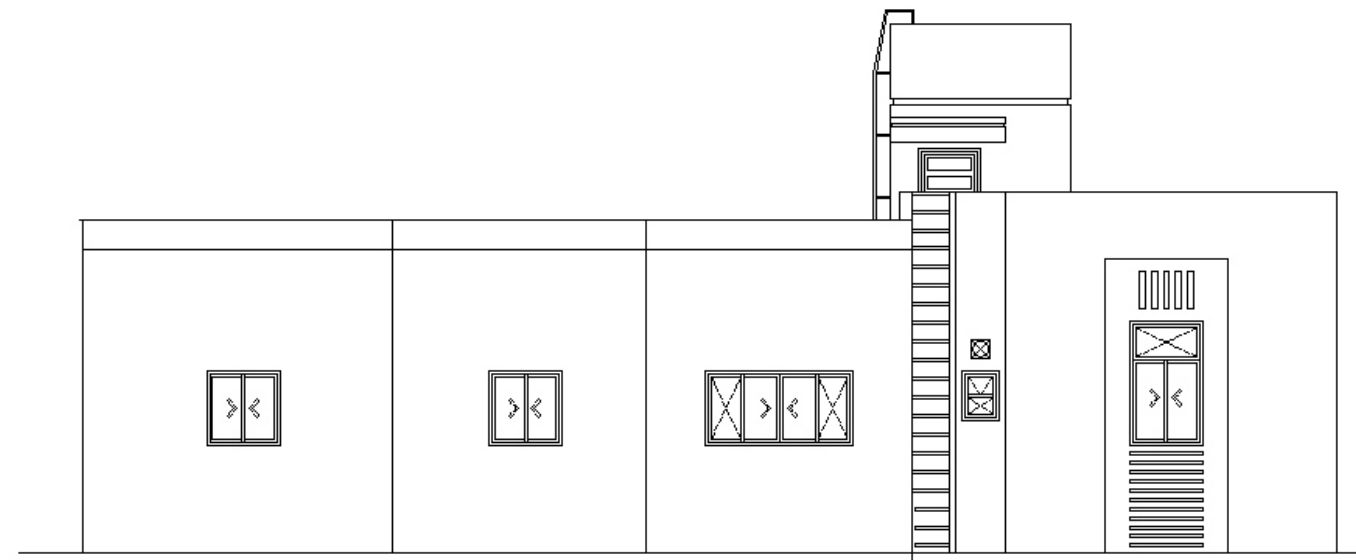
الواجهه الجانبية
