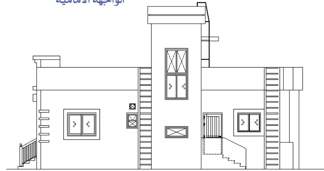
الواجهة الجانبية
